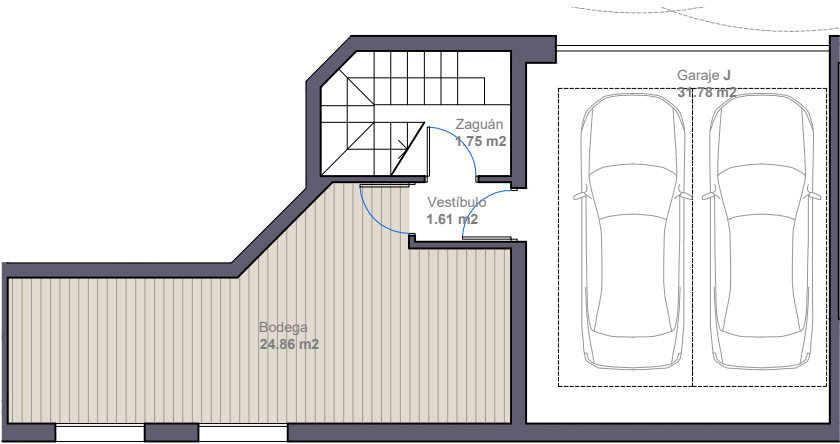
DETALLE BODEGA SEMISÓTANO E.1/200
