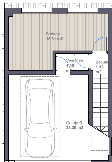
DETALLE BODEGA SEMISÓTANO E.1/200
