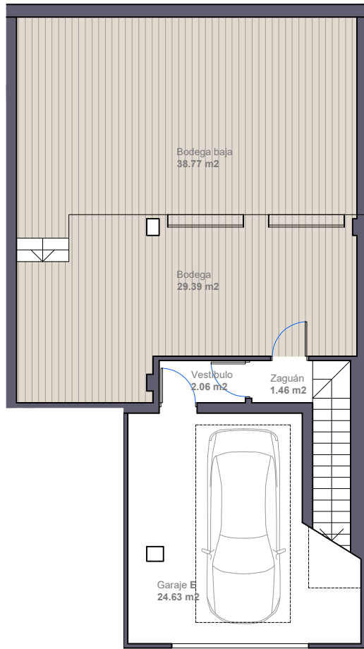
DETALLE BODEGA SEMISÓTANO E.1/200
