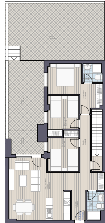
DETALLE TERRAZA E.1/200
