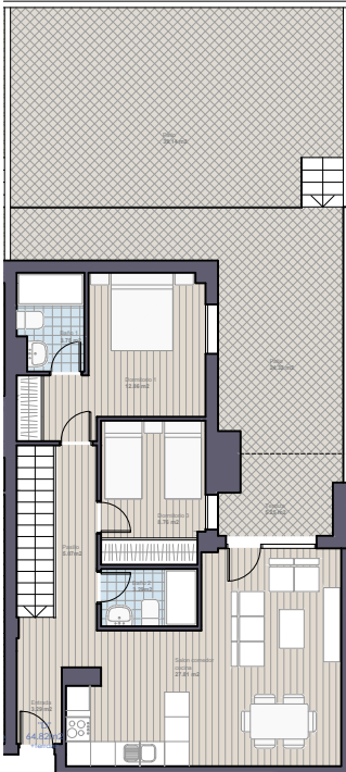
DETALLE TERRAZA E.1/200
