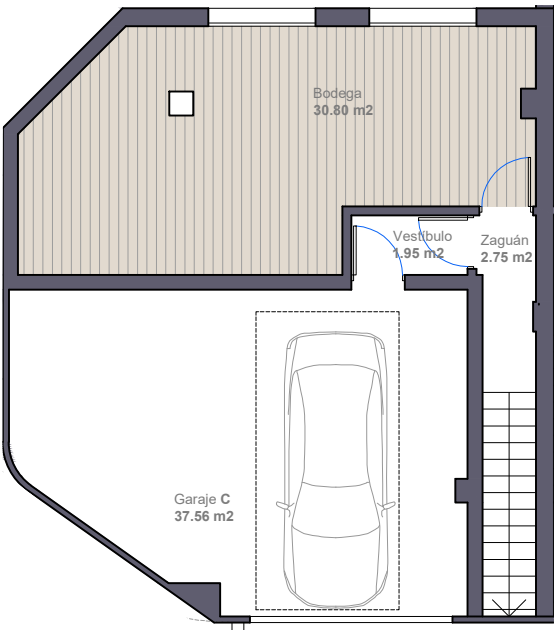
DETALLE BODEGA SEMISÓTANO E.1/200
