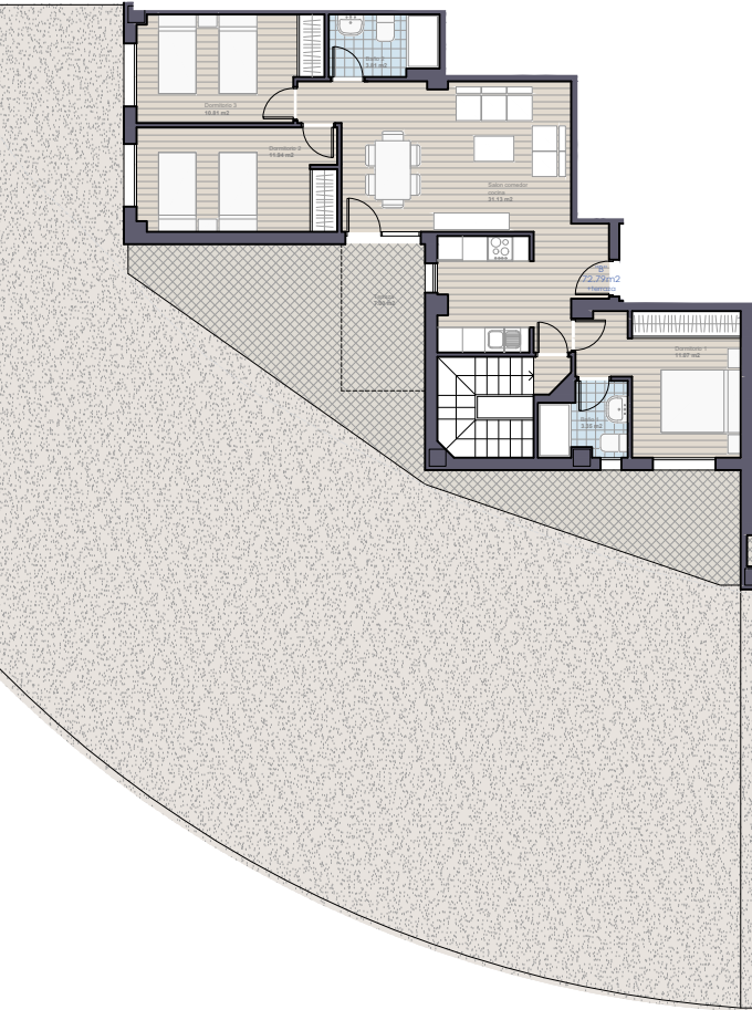
DETALLE TERRAZA y ZONA DE USO PRIVATIVO E.1/200
