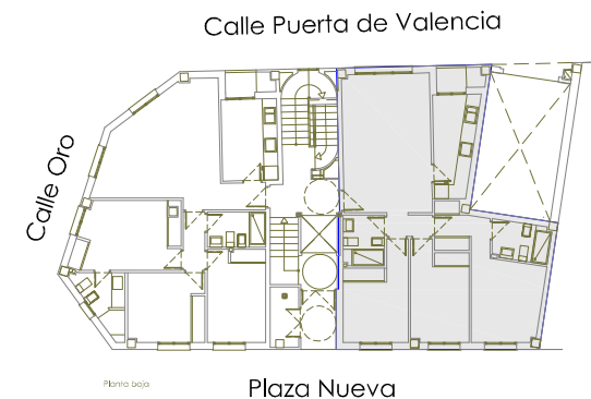
VIVIENDA TIPO B planta baja Superficie útil: 76,55m 2 e 1/50
