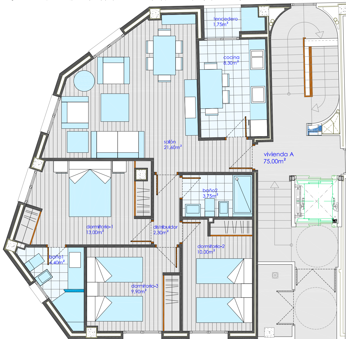
VIVIENDA TIPO A planta baja Superficie útil: 75,00m 2 e 1/50
