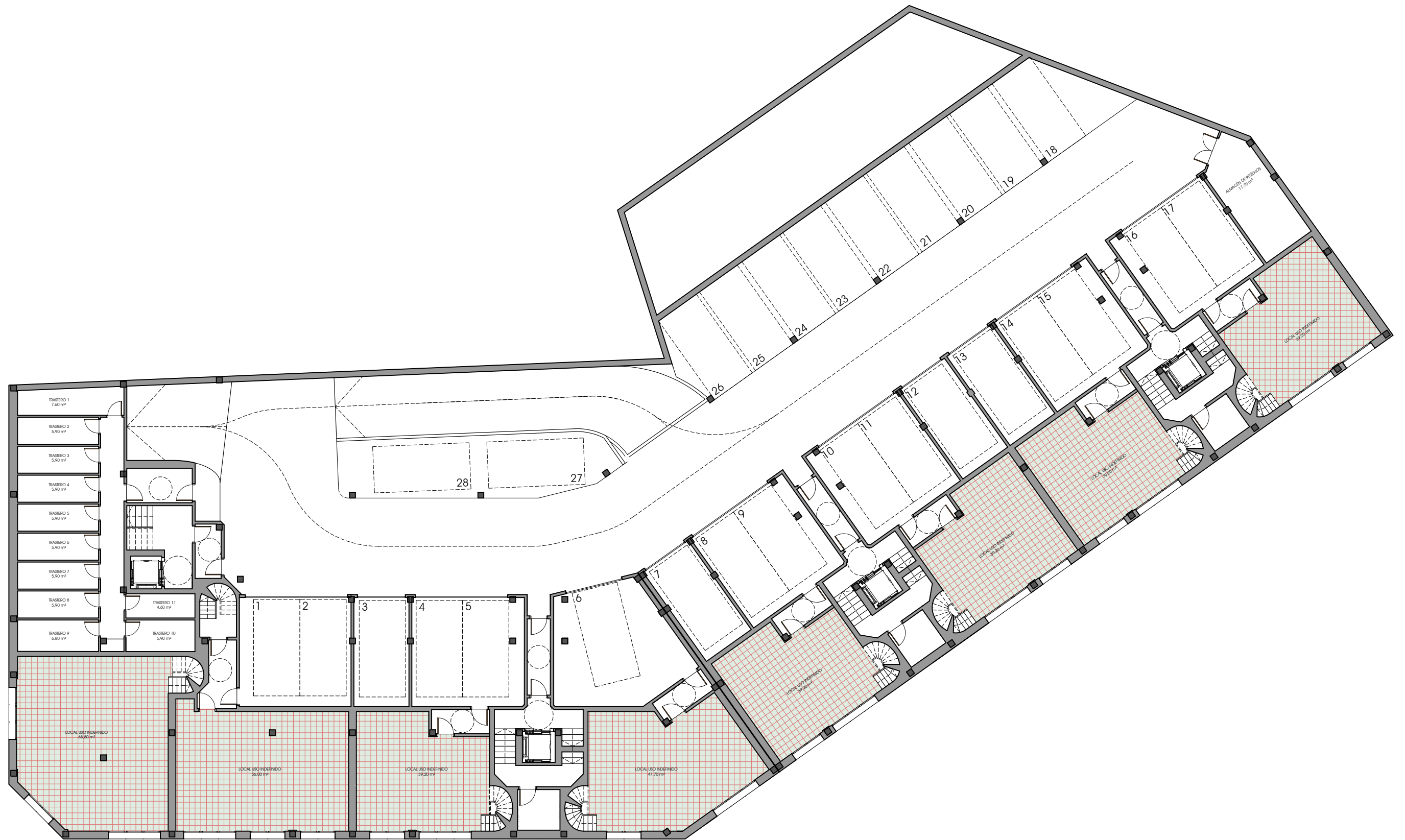
PLANTA SÓTANO -1
